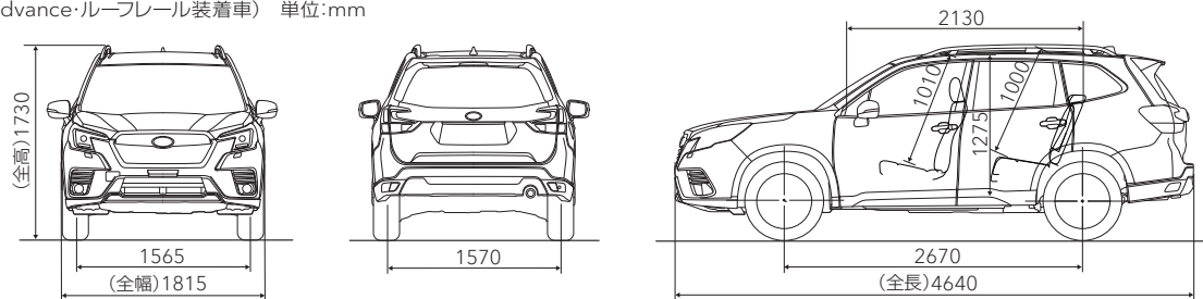
3面図(Advance・ルーフレール装着車) 単位:mm
