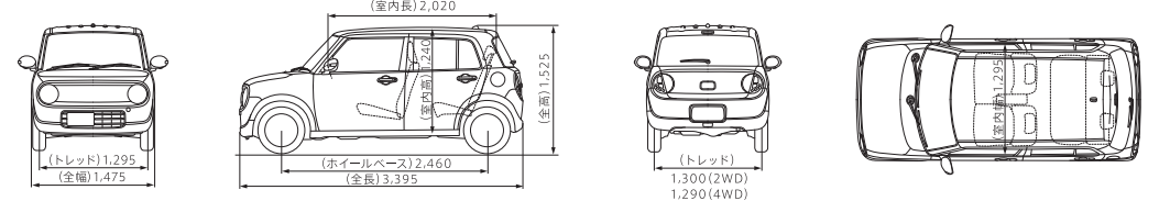
寸法図(X) 単位: mm
