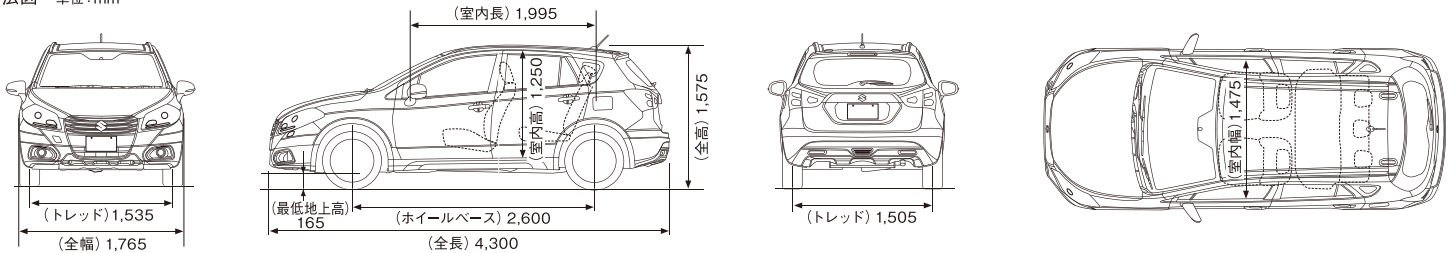
寸法図 単位: mm
