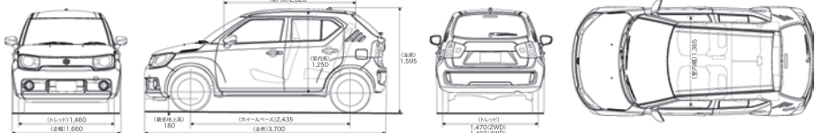
寸法図(HYBRID MZ) 単位:mm
